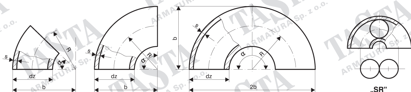
Kolana wg ANSI B16.9 typ SR
